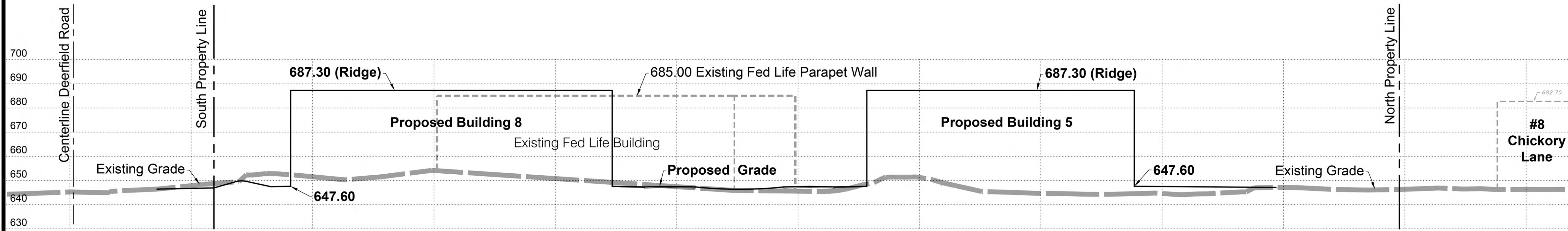
Section A-A Scale: 1" = 20'
